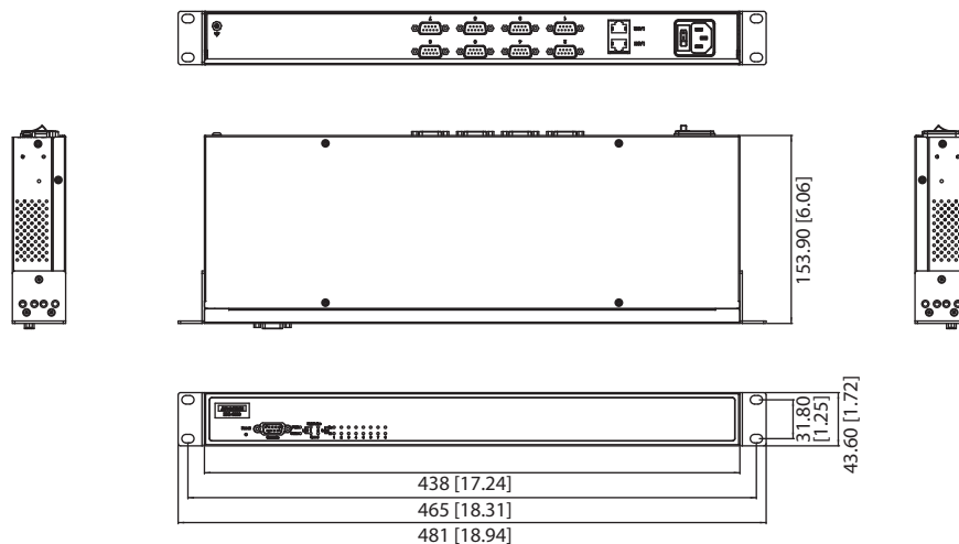
EKI-1528-I1A
